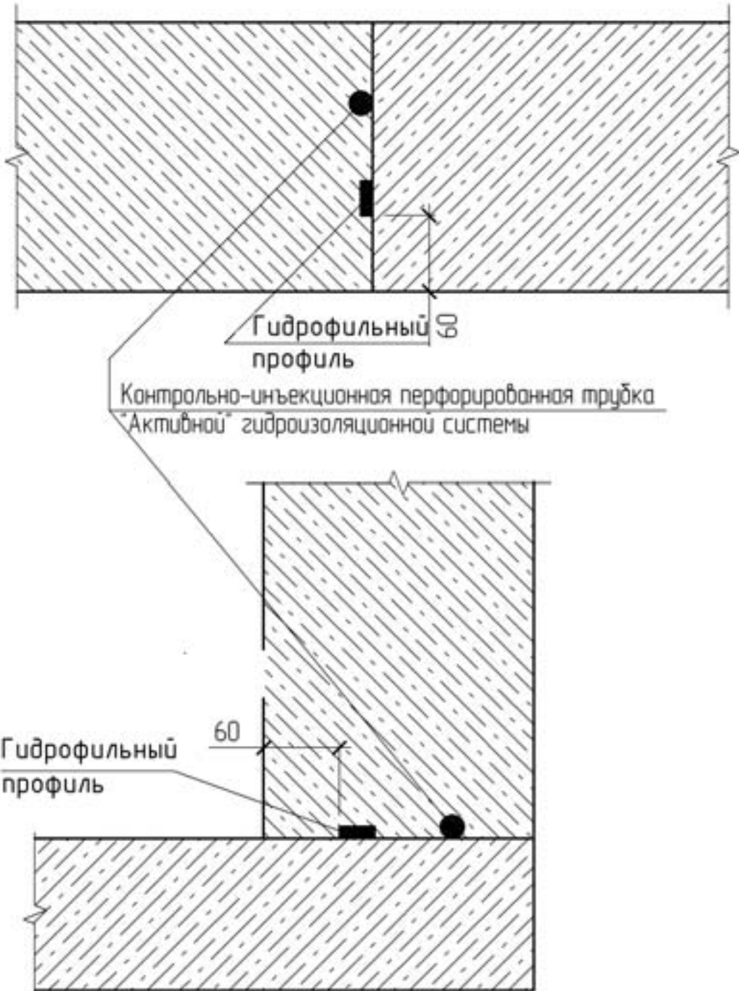
Узел активной гидроизоляционной системы холодного шва
