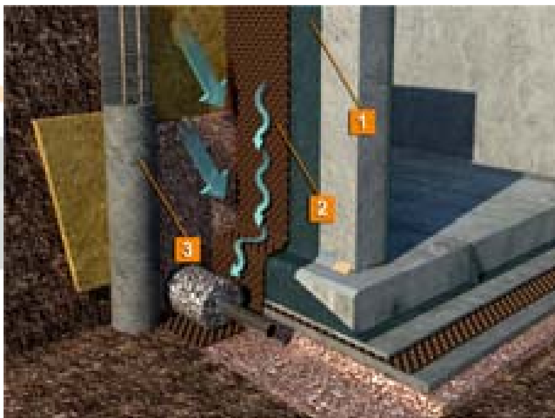
1 - Гидроматик, Гидроматик Ф, Гидроматик Флекс 2 - Дренажное полотно 3 - Стена в грунте
